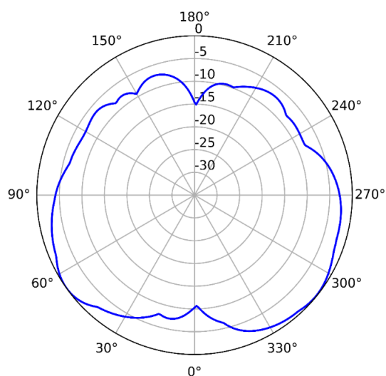
2.4GHz (Vertical)
