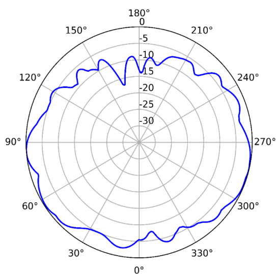
5GHz (Vertical)
