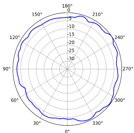
5GHz (Horizontal)
